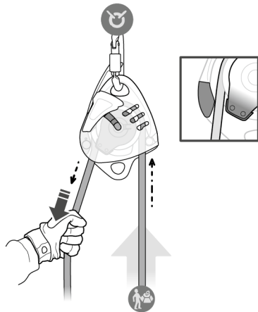
Hauling Hissage
